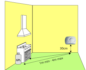
Fig.2: Rivelazione gas GPL
